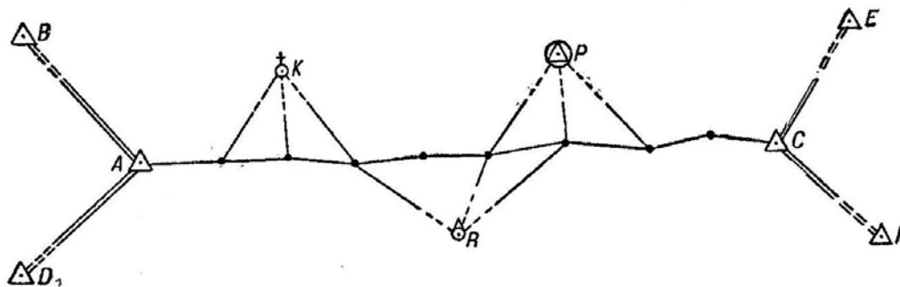
Рис. 61. Теодолітний хід між вихідними пунктами
