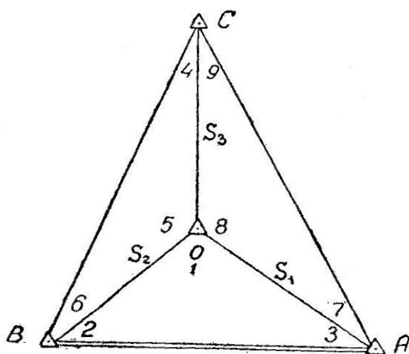
Рис. 161. Вільна мережа тріангуляції
