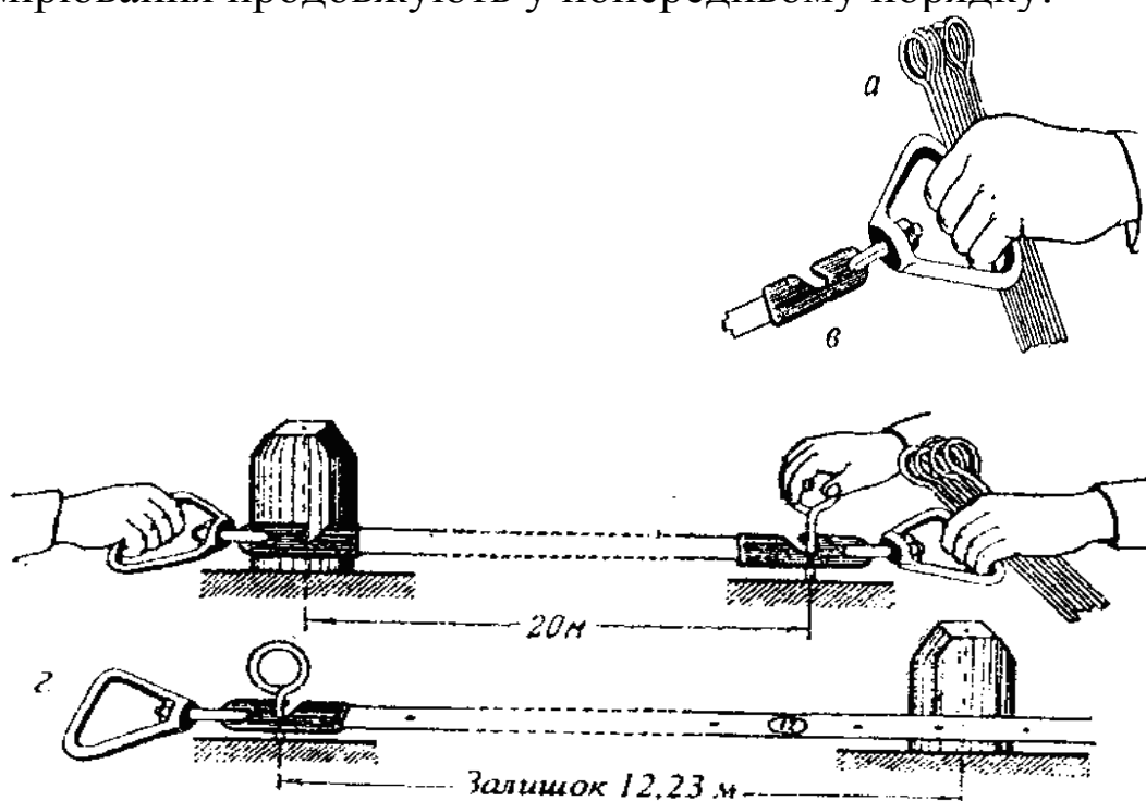
Рис. 40. Вимірювання ліній
