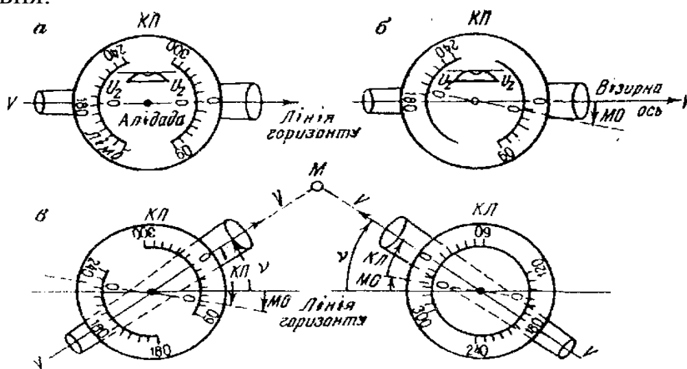
Рис. 54. Вертикальний круг
