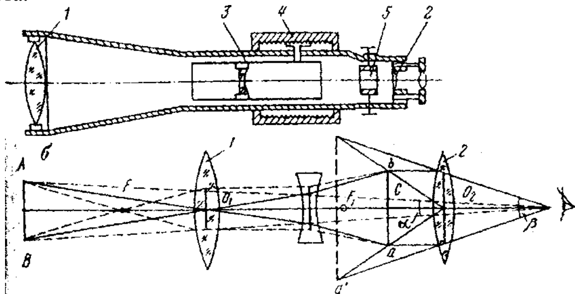
Рис. 49. Зорова труба
