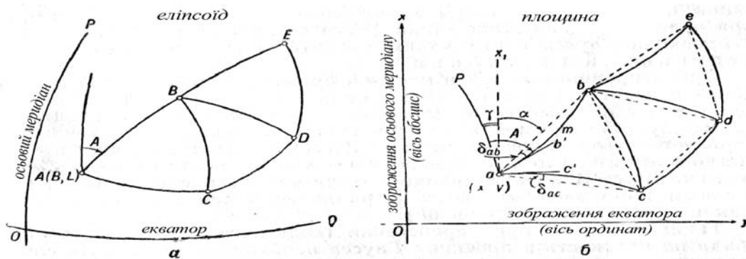
Рис.176. Зображення геодезичної мережі
