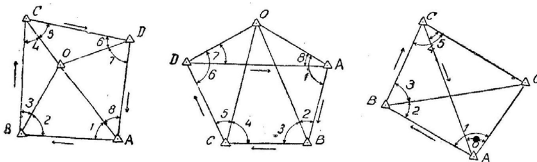
Рис. 162, 163, 164. Фігури триангуляцій
