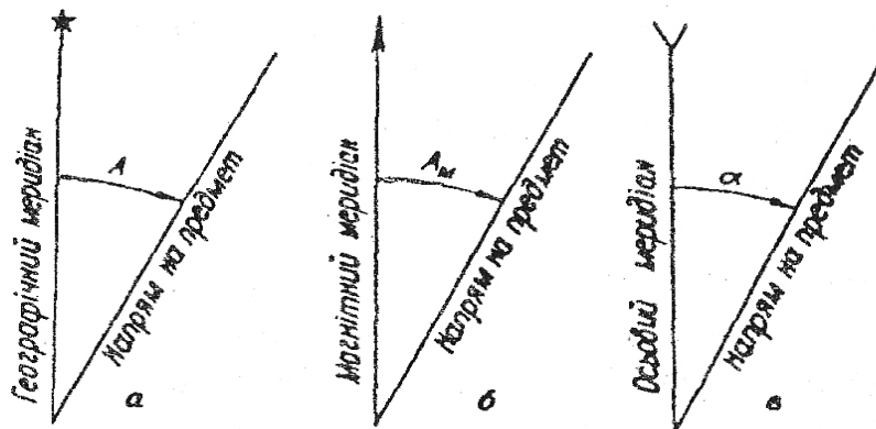
Рис. 17. Кути орієнтування
