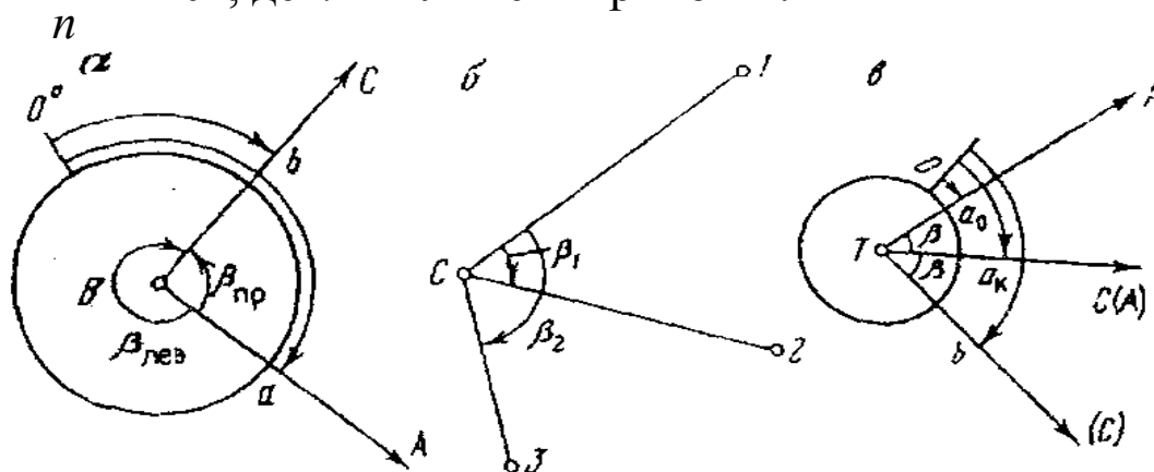
Рис. 57. Способи вимірювання горизонтальних кутів
