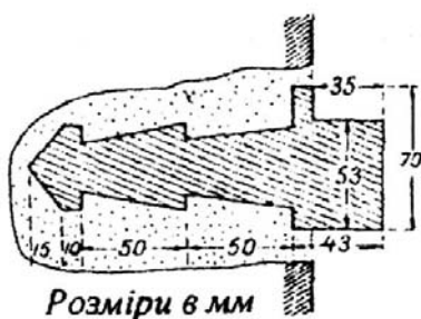
Рис. 86. Стінна марка
