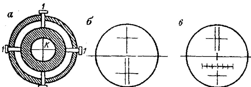
Рис. 50. Сітка ниток зорової труби:
