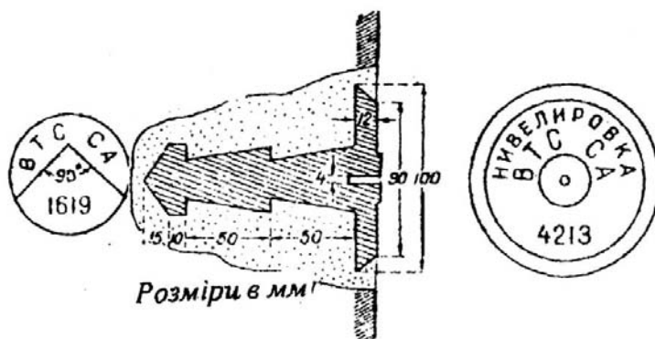
Рис. 87. Стінний репер
