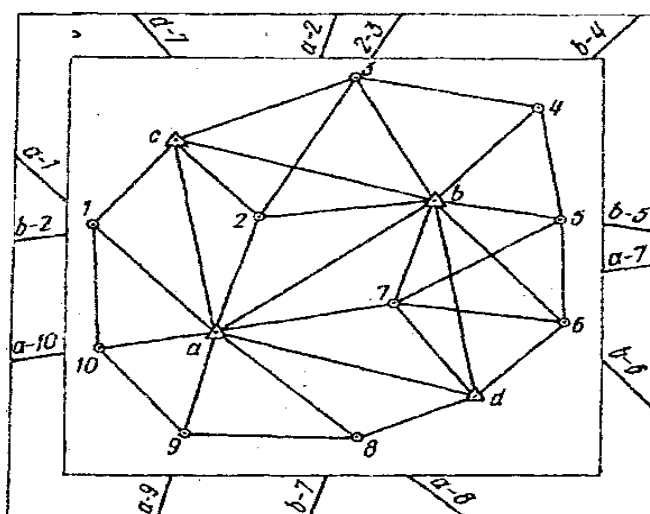
Рис. 117. Визначення положення точок геометричної сітки
