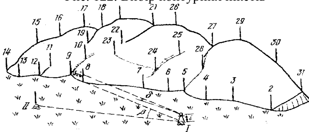
Рис. 122. Вибір контурних пікетів
