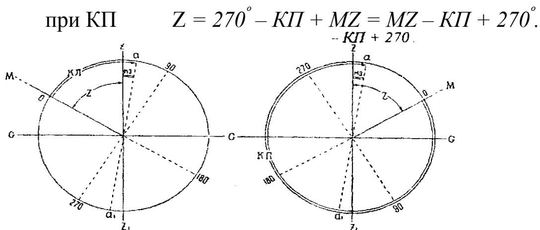
Рис. 56. До обчислення вертикальних кутів, вимірних теодолітом ТБ-1
