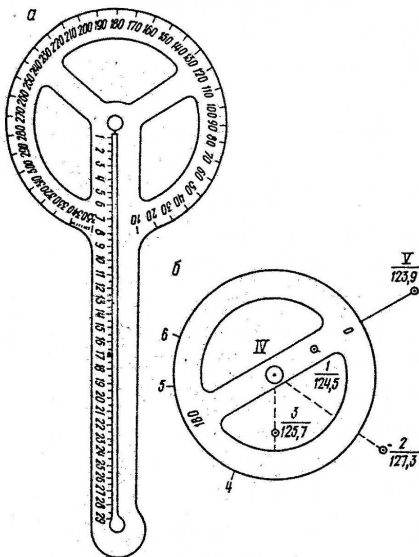
Рис. 126. Тахеограф
