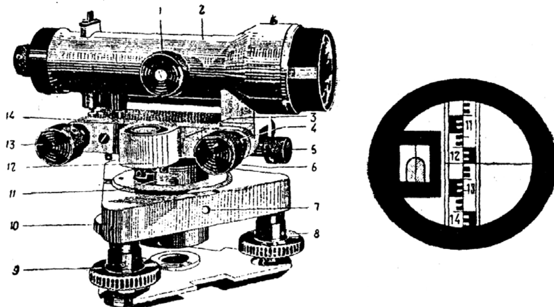
Рис. 90. Нівелір Н-3 Рис. 91. Поле зору зорової труби
