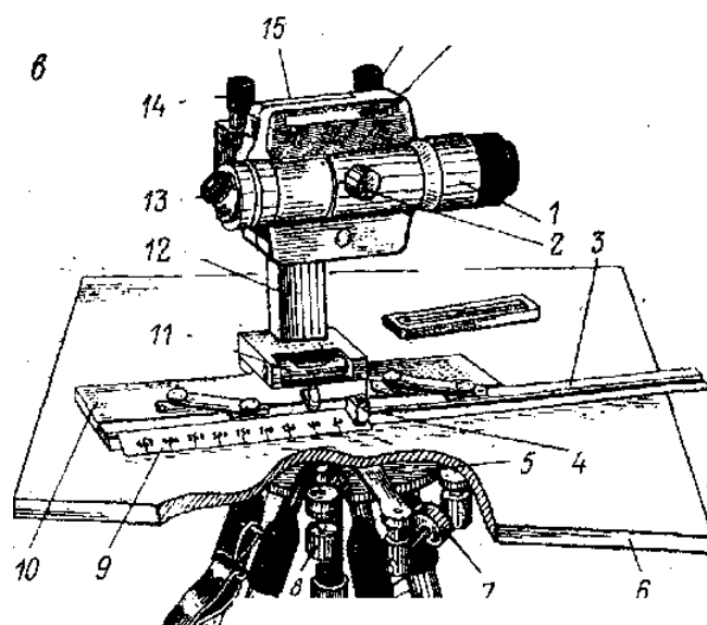
Рис. 112. Кіпрегелі a – КА-2; б – поле зору труби КА-2; в – КН; г – поле зору труби КН
