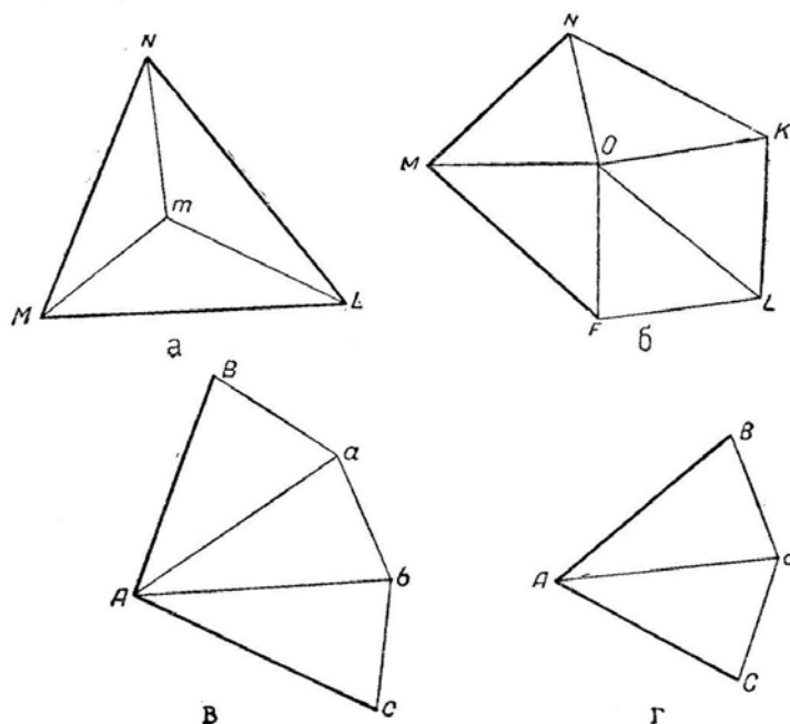
Рис. 130. Типові фігури при вставці окремих пунктів: a – вставка пункту в трикутник; б – центральна система; в – вставка двох пунктів у кут; г – вставка одного пункту в кут
