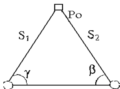
Рис. 135. Розшук пункту за двома ОРП, що збереглися
