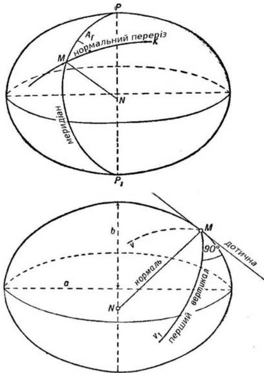
Рис. 6. Геодезичний азимут
