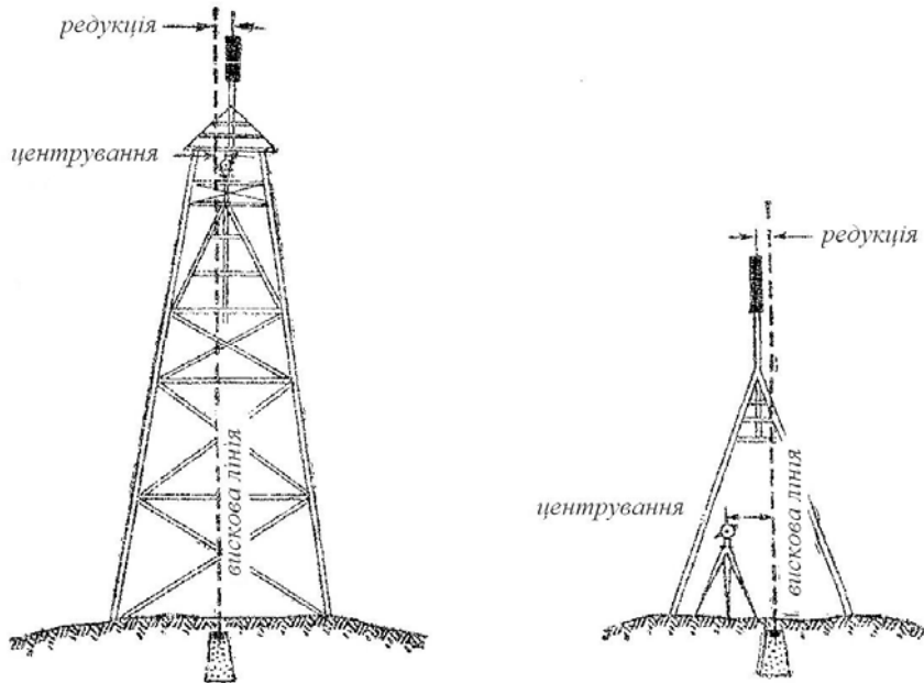
Рис. 140. Позацентроване положення теодоліта і візирної цілі
