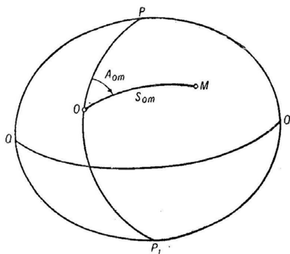
Рис. 13. Сферичні полярні координати точки M ( S_{om}, A_{om} )
