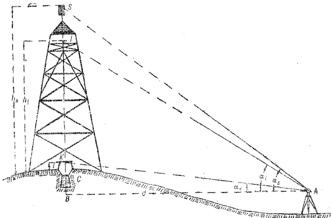
Рис. 149. Визначення висоти знака аналітичним способом
