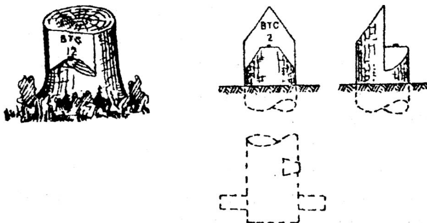
Рис. 89. Тимчасові репери
