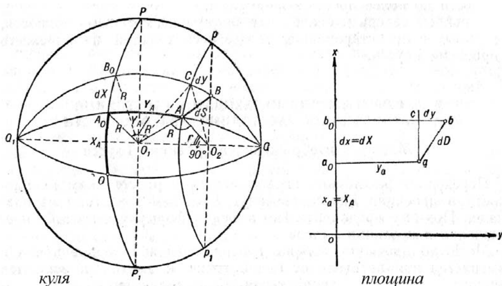
Рис. 177. Масштаб зображення
