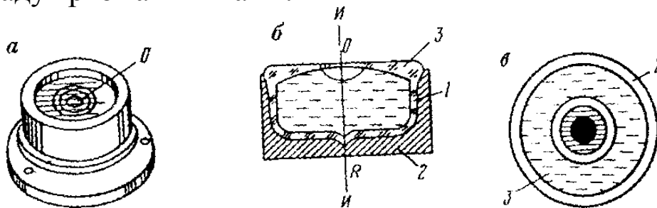
Рис. 53. Круглий рівень:
