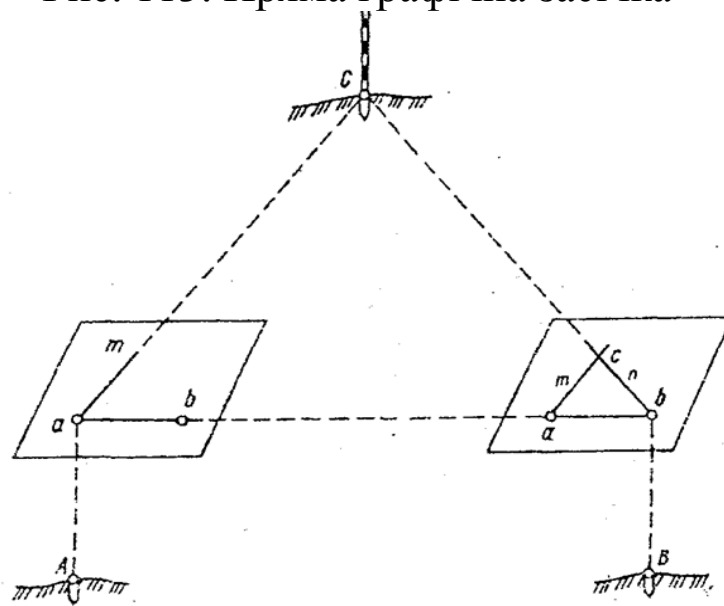
Рис. 114. Зворотна графічна засічка
